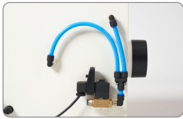
자동에어분사장치
